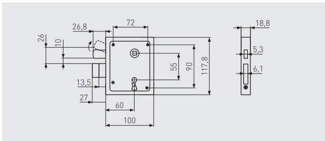
AUFSCHRAUBSCHLOSS ASS SF BB
