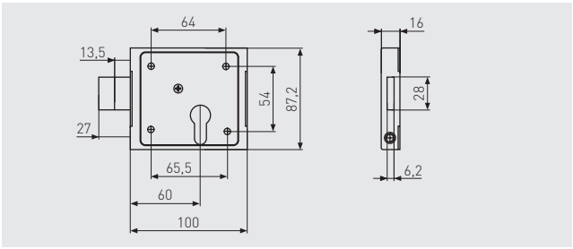
AUFSCHRAUBSCHLOSS ASS HF PZ
