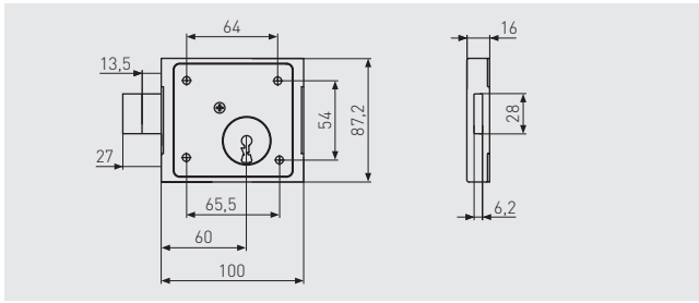
AUFSCHRAUBSCHLOSS ASS HF BB
