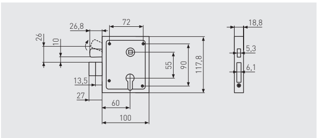
AUFSCHRAUBSCHLOSS ASS SF PZ
