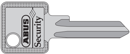
10023 Rohling Türzylinder C73, C83, K82 Messing R, eckiger Schlüsselkopf
