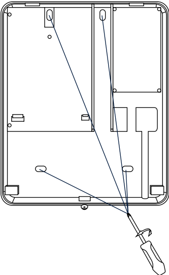
Behuizing monteren 3
