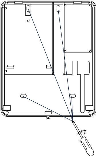
Monter hus
