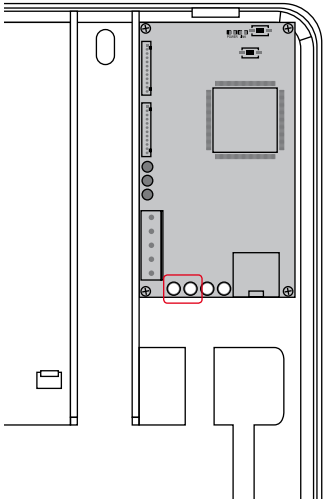
Netadapter aan de Secvest monteren 1
