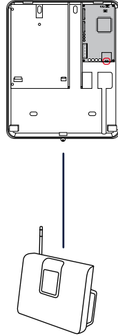
LAN-Kabel anstecken oder Secvest IP mit Router verbinden
