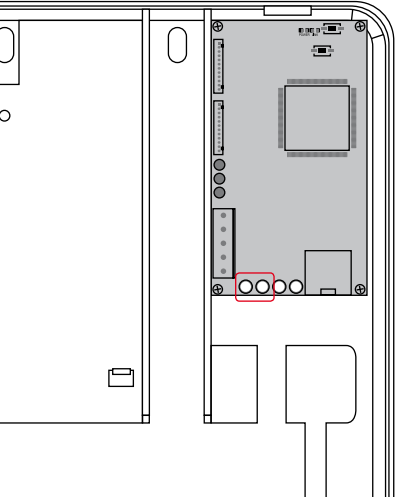
Netzteilkabel an Secvest montieren
